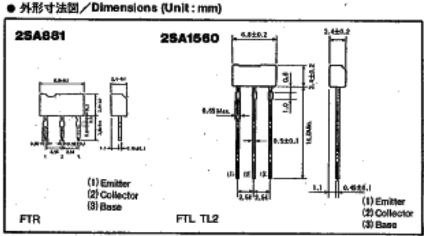
注: FTLの外形仕様については, TL3/4タイプも用意しています (p.38参照)。
