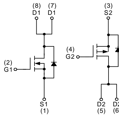
N-Channel MOSFET P-Channel MOSFET
