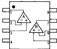
NJM4560D/M/E
